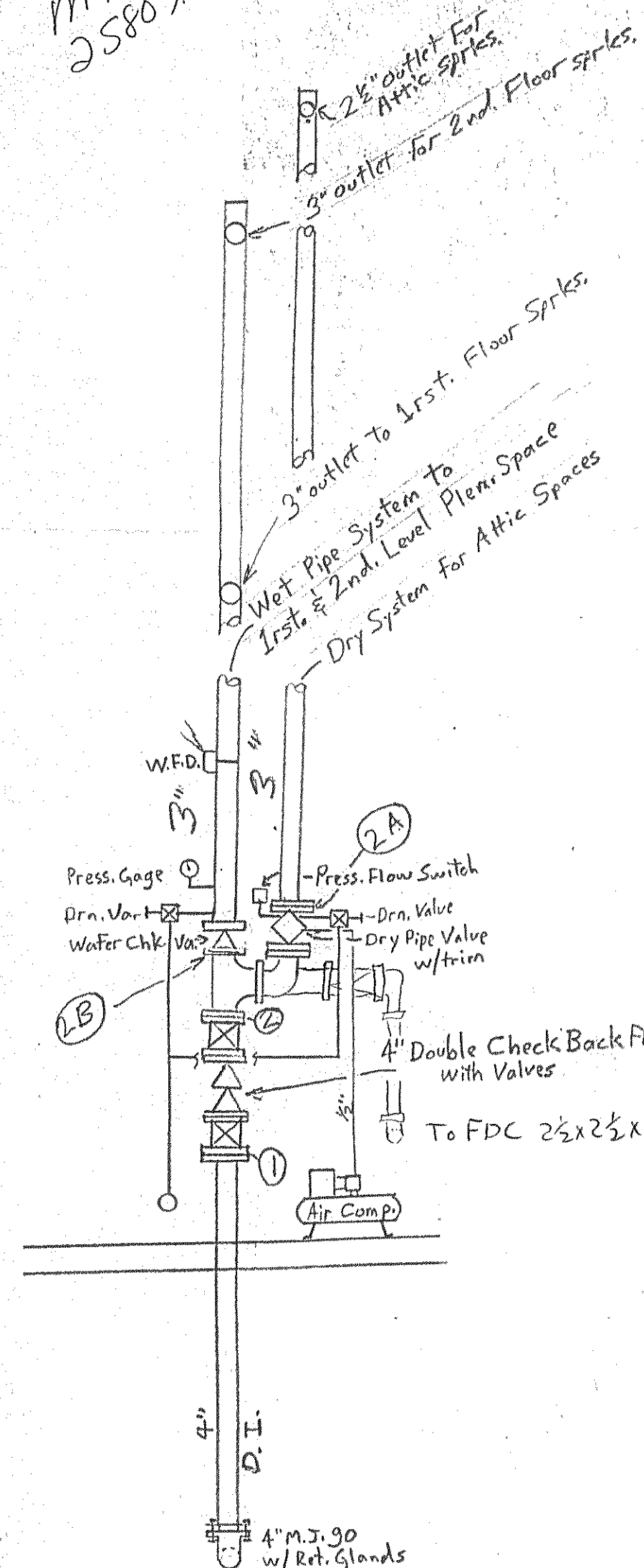
RISER DETAIL N.T.S.
